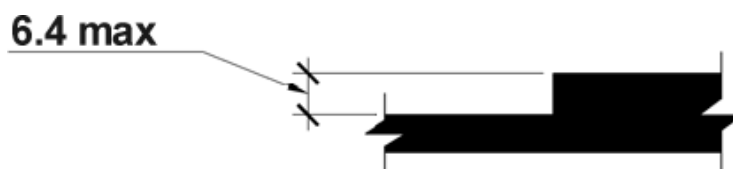
Figur 2 Loddrett nivåendring
