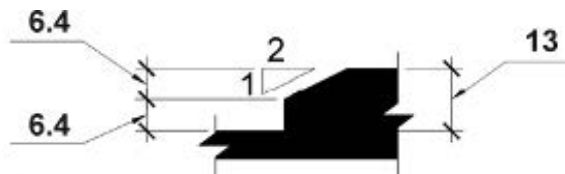
Figur 3 Skrå nivåendring
