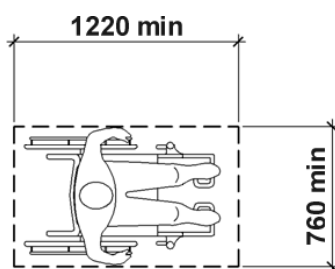
Figur 4 Fritt areal
